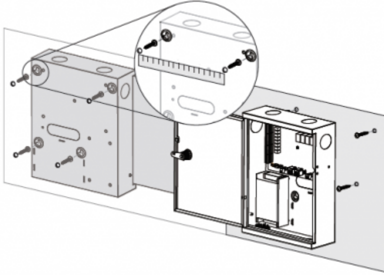
图3-3 安装示意图
