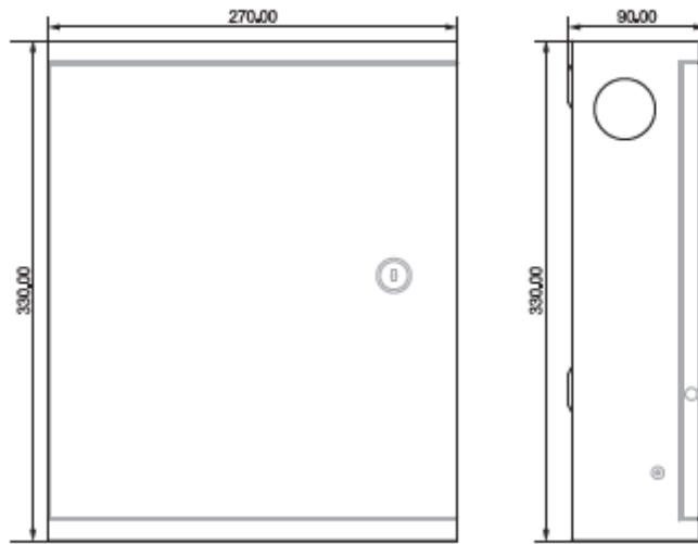
图1-1 外观尺寸
